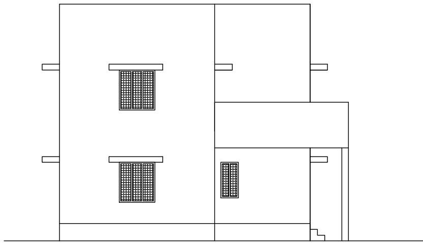
ELEVATION
