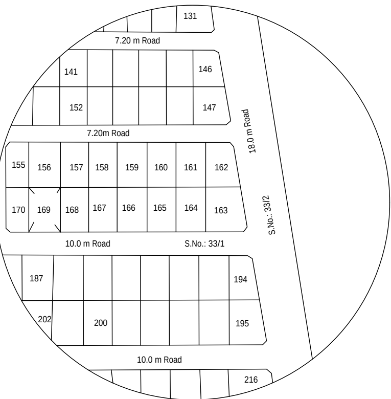
LAY-OUT
