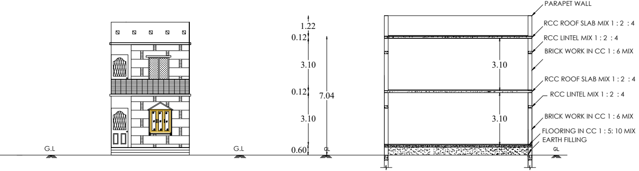
ELEVATION
