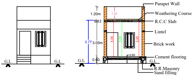
ELEVATION
