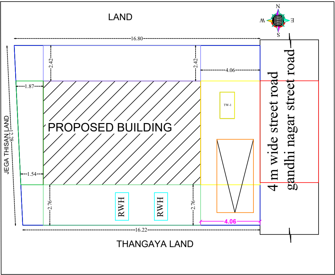
SITE PLAN 1:100 SCALE
