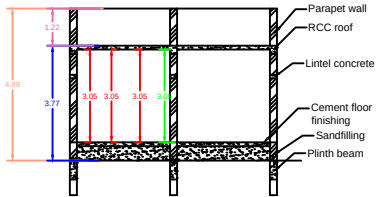
SECTION - AB
