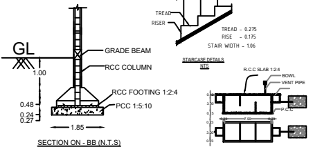
SECTION ON - BB (N.T.S.)
