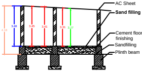
SECTION - AB
