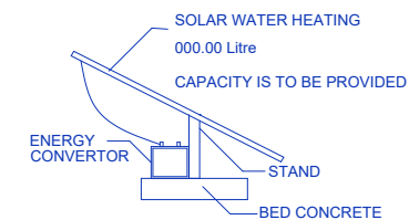
LONGITUDINAL SECTION
