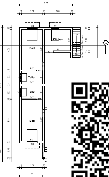
GROUND F1
