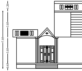
ELEVATION
