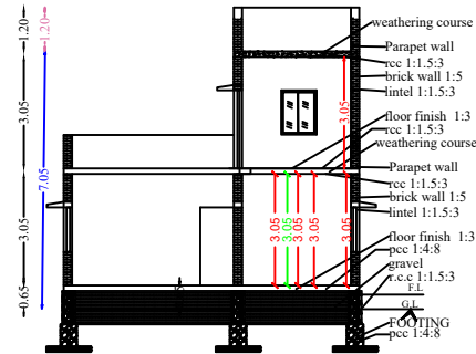
SECTION A-A & B-B
