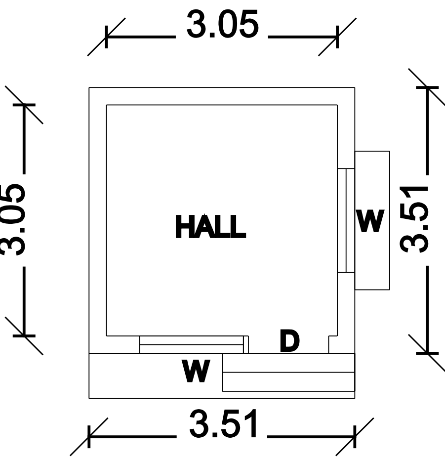
G.F PLAN
