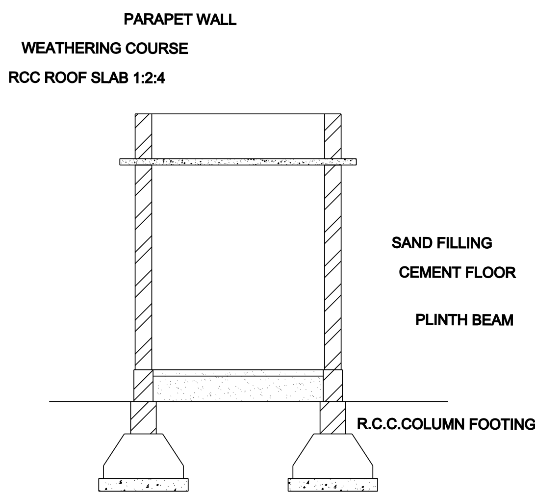
SECTION - AB
