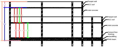
SECTION - AB
