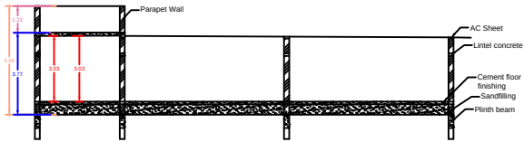
SECTION - AB
