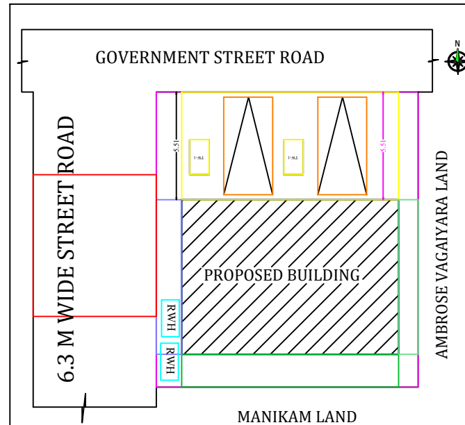
SITE PLAN 1:100 SCALE
