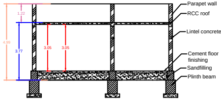
SECTION - AB
