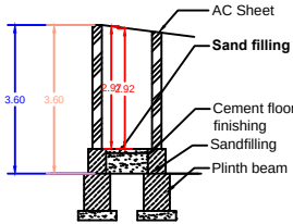
SECTION - AB
