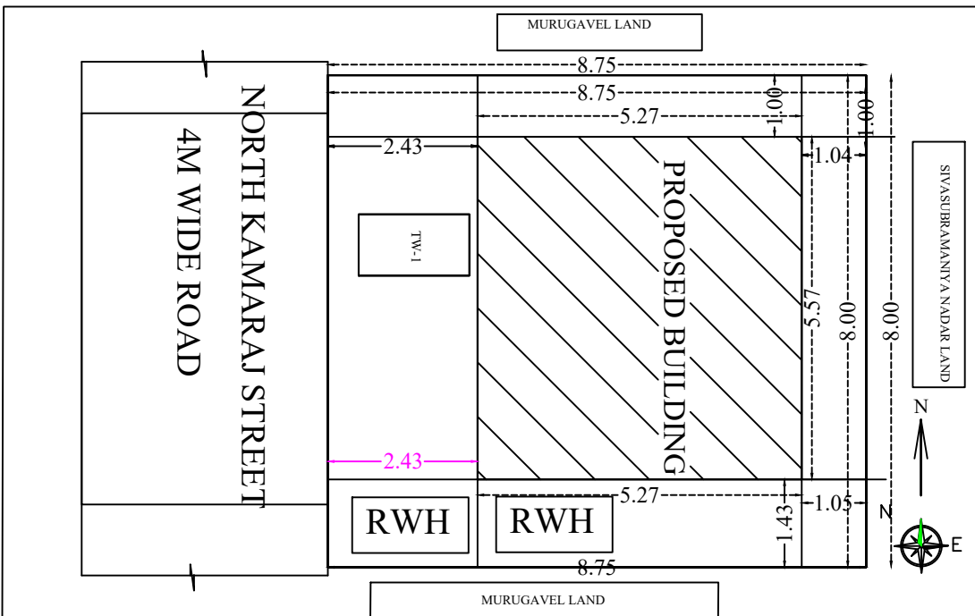
SITE PLAN 1:100 SCALE
