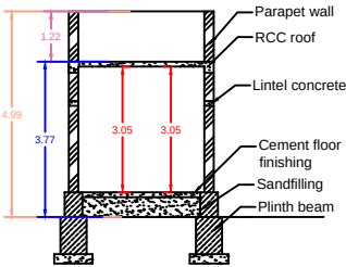
SECTION - AB
