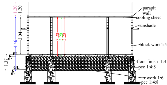
SECTIONN A-A
