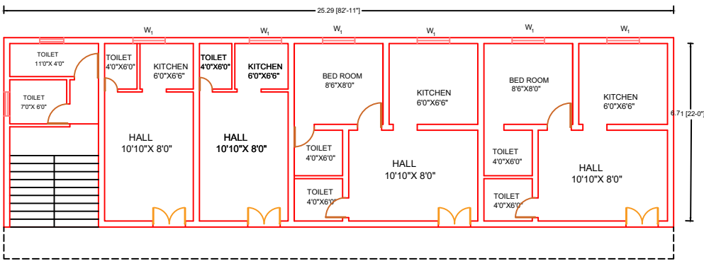
F.F. PLAN
