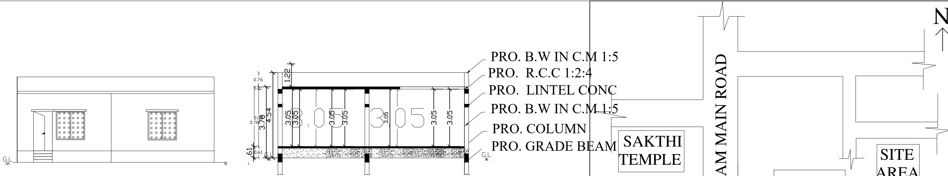
ELEVATION
