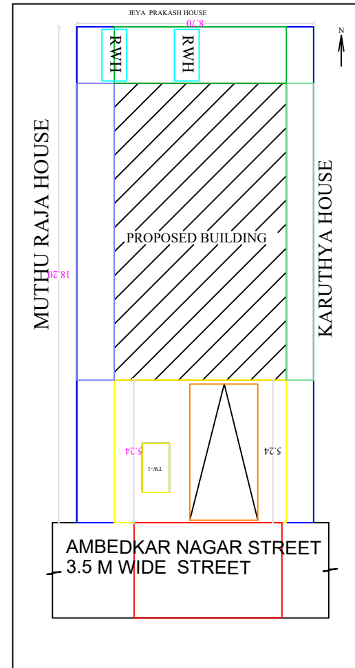
SITE PLAN 1:100 SCALE
