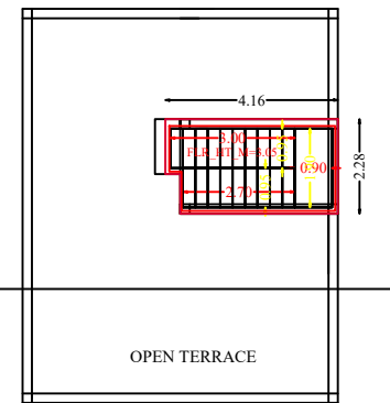
F.F PLAN
