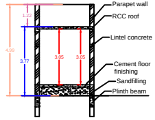
SECTION - AB
