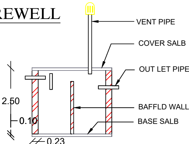
SECTION ON X - Y
