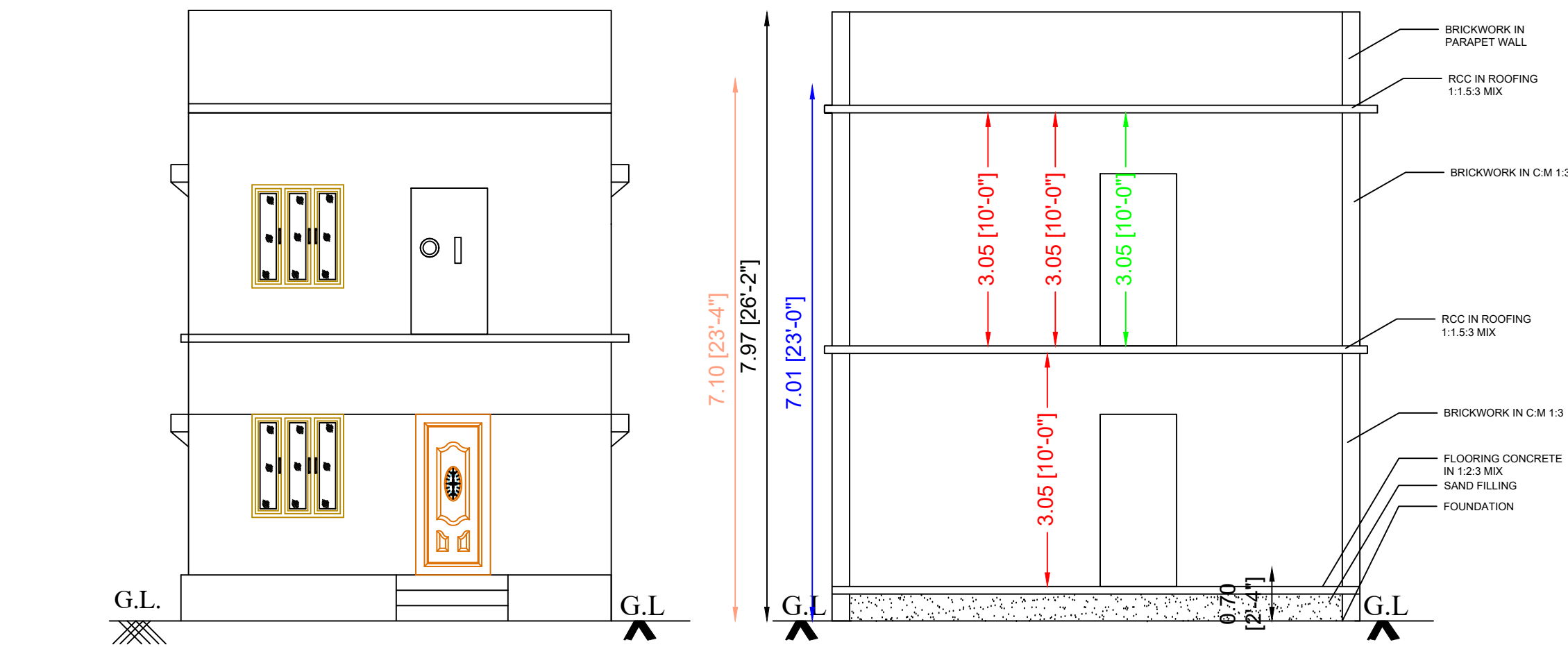
ELEVATION
