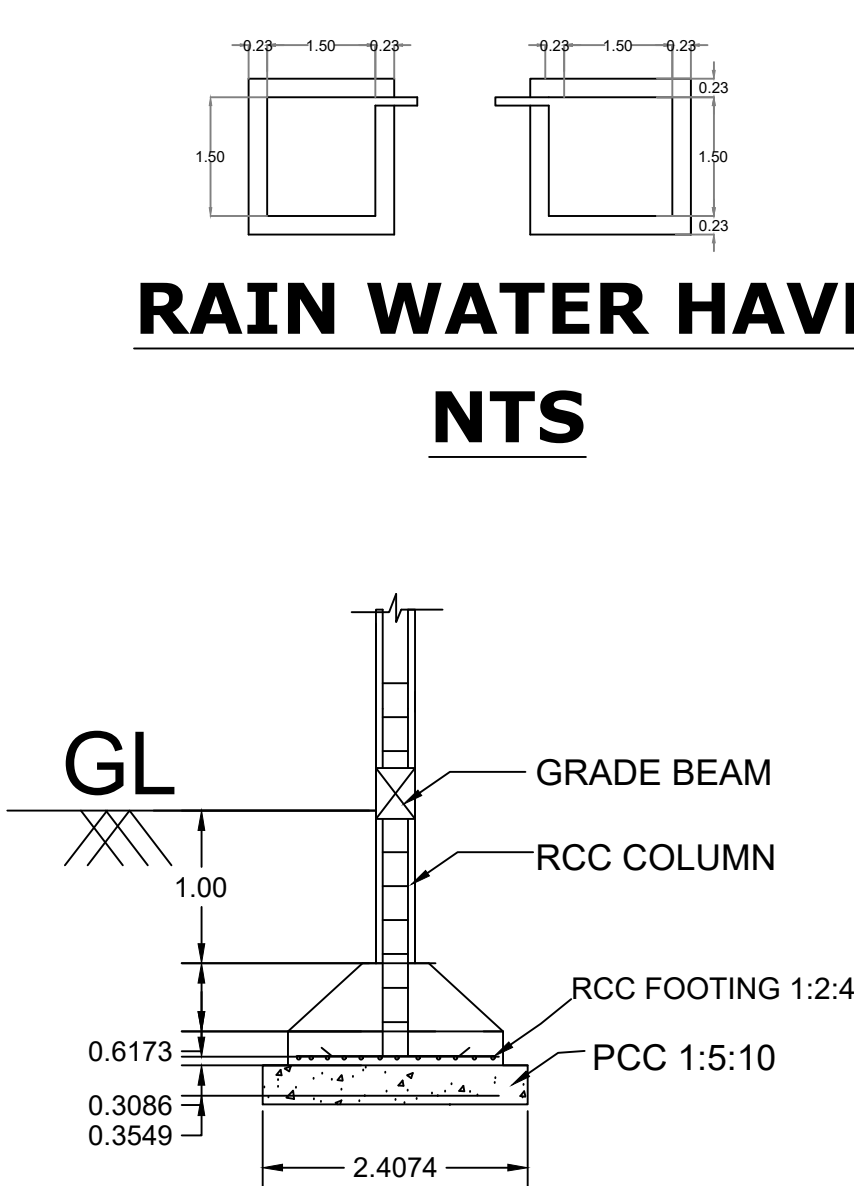
SECTION ON - BB (N.T.S)
