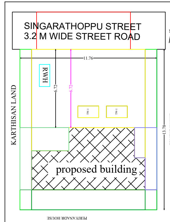
SITE PLAN 1:100 SCALE
