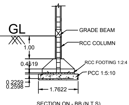
SECTION ON - BB (N.T.S)
