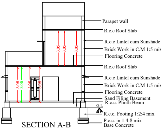
SECTION A-B
