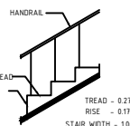
STAIRCASE DET.
