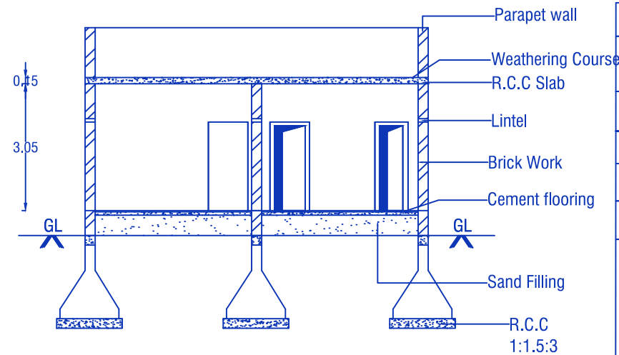
SECTION ON'AB'
