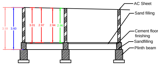
SECTION - AB
