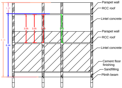
SECTION - AB
