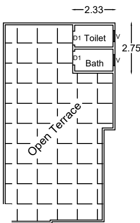
RO.F.F PLAN
