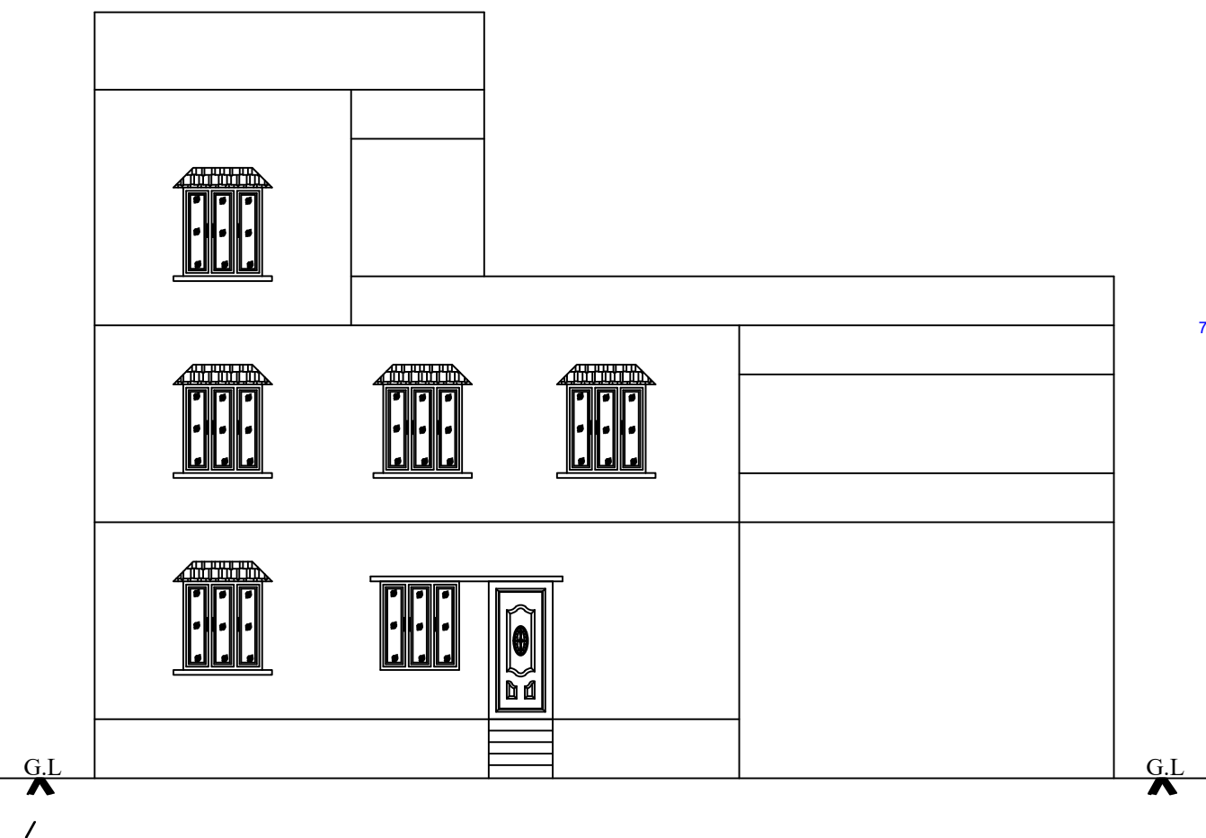
ELEVATION
