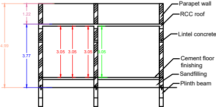
SECTION - AB
