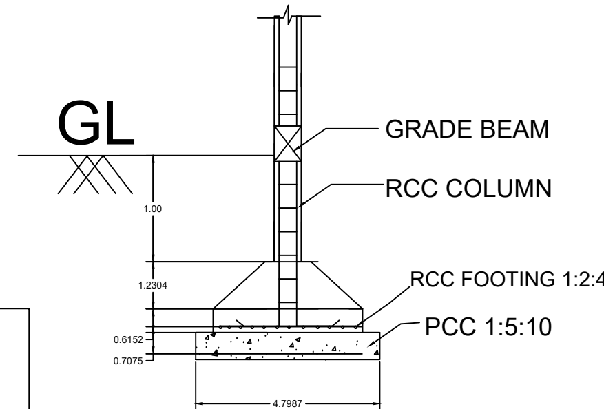
SECTION ON - BB (N.T.S)
