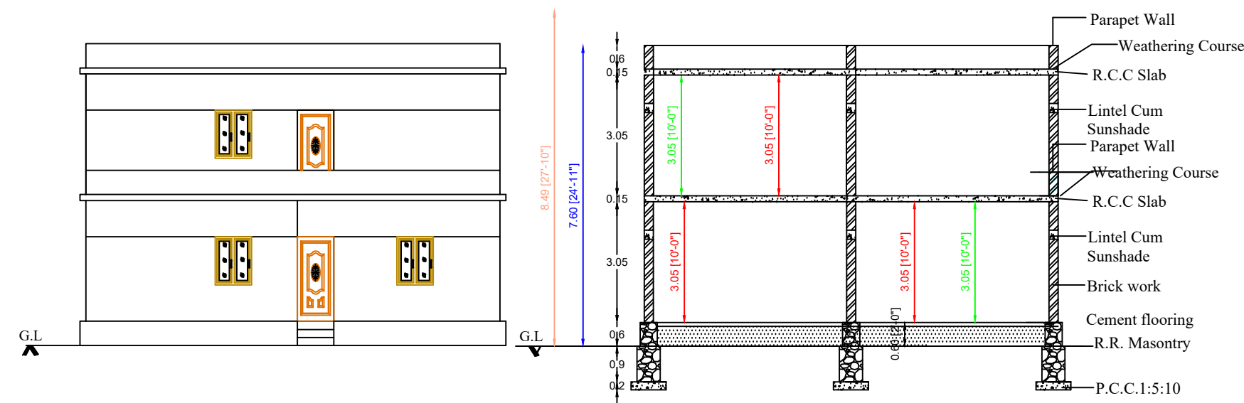
ELEVATION
