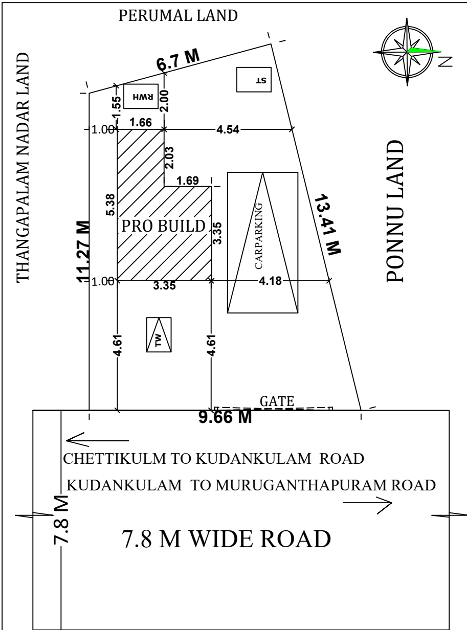
SITE PLAN 1:100 SCALE
