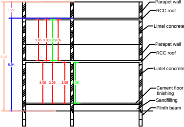
SECTION - AB
