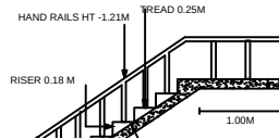
SECTION - AB
