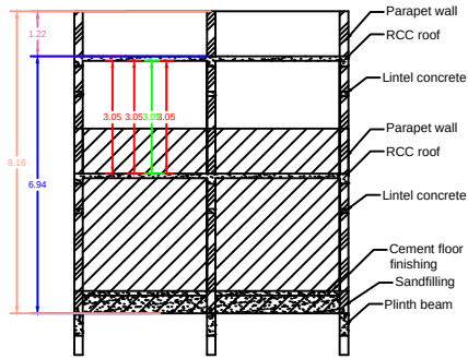
SECTION - AB
