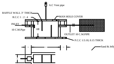
SEPTIC TAN
