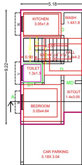
G.F PLAN
