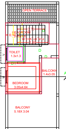
F.F PLAN
