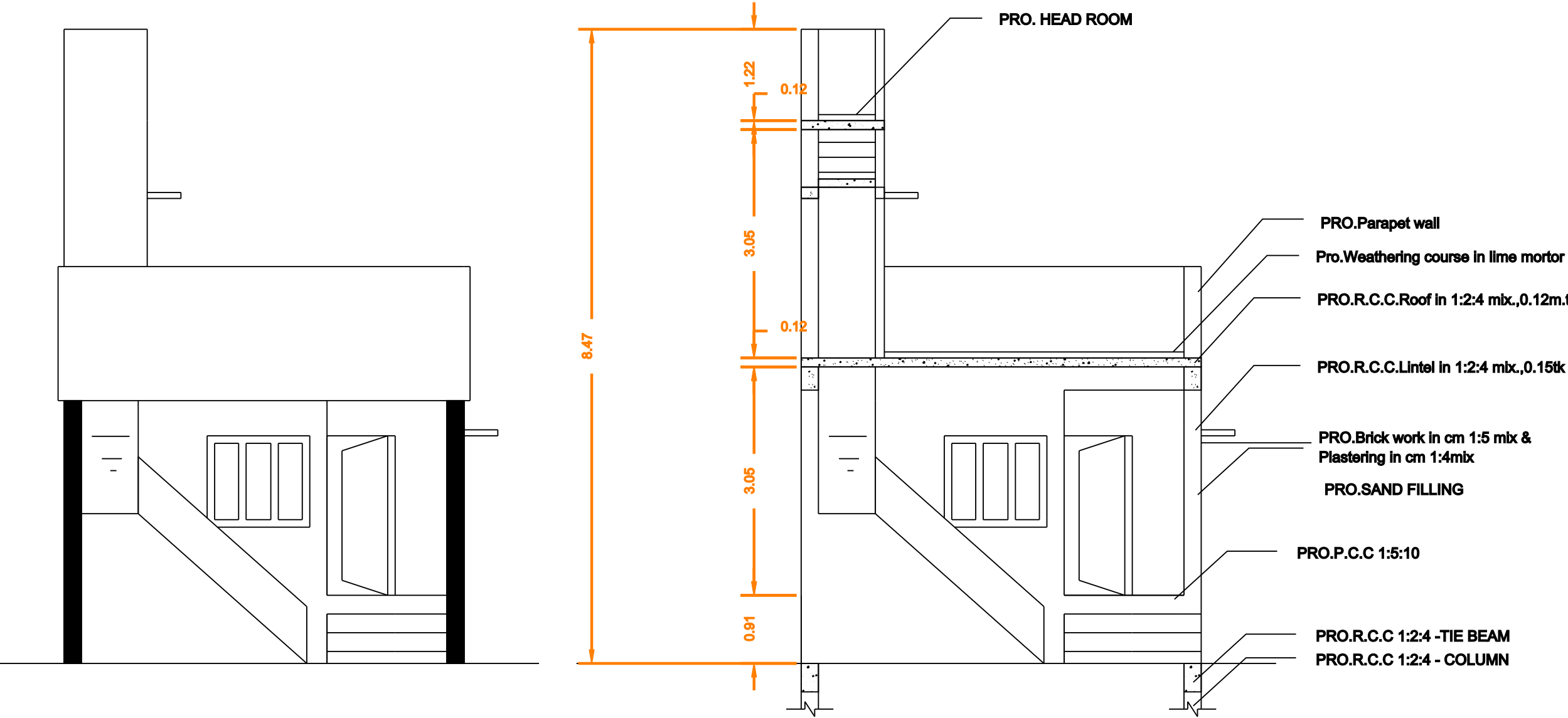
ELEVATION
