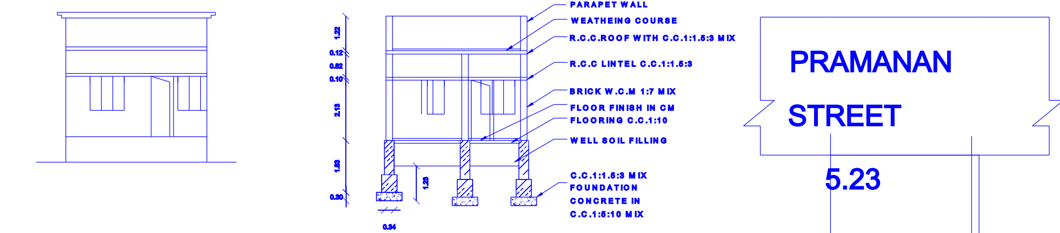
ELEVATION
