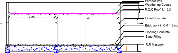
SECTION-E1E1
