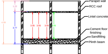
SECTION - AB
