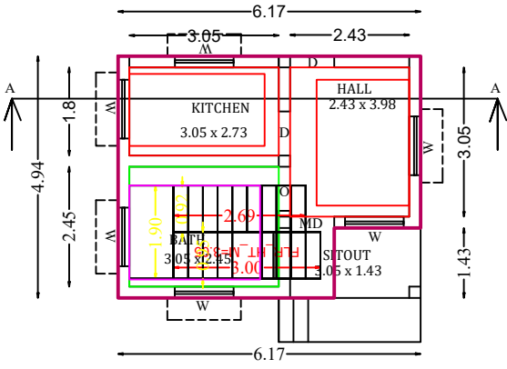
F.F PLAN
