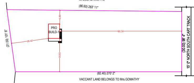
SITE PLAN.SCALE :1:400
