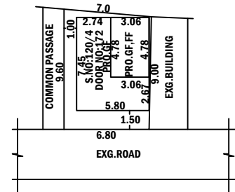
SITE PLAN (SCALE 1:200)
